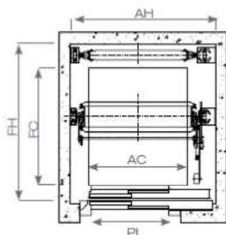
Plano de planta
